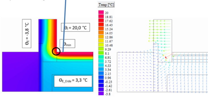
Temperaturverteilung und Wärmefluss
