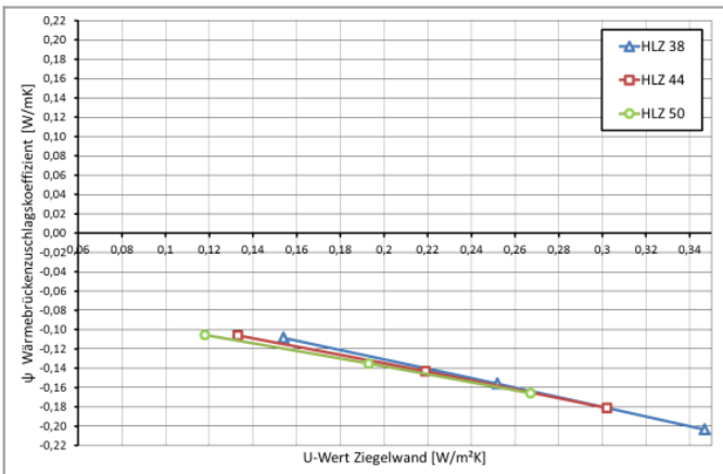
Linearer Wärmebrückenzuschlagskoeffizient \psi
